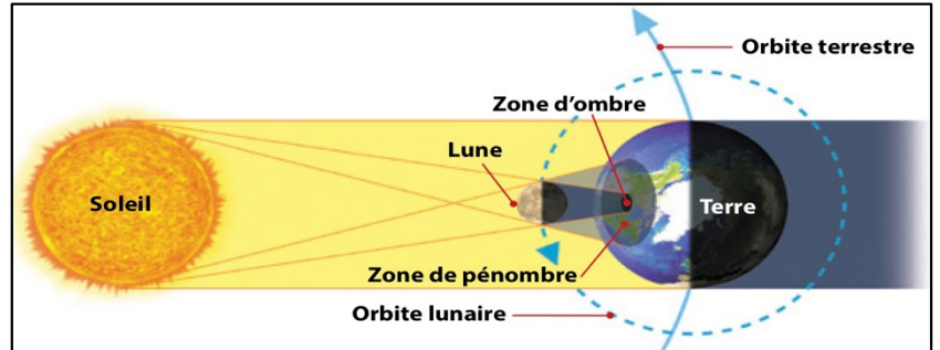
Schéma # 1 : La lune entre le soleil et la Terre. Crédit : Éditions CEC, 2019.
